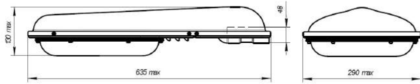
Светильник
