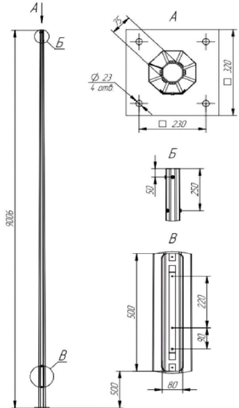
Опора
